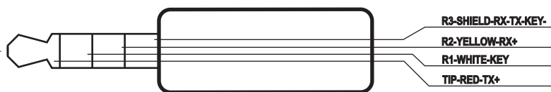
Straight: PN R3CBLAUD (Kobiconn 172-7435)
